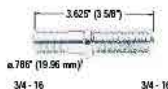
5105-R
