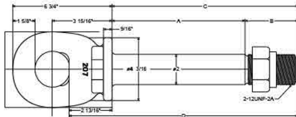
PRE207S ARGOLLA DE ARRASTRE CON BARRA GIRATORIA
