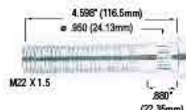
9501-R
