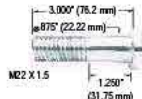
500-R
