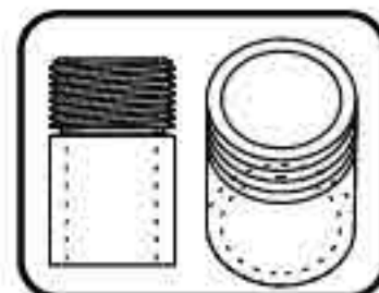
BOCA DE CARGA DE 3 1/2" DE DIAMETRO POR 3 1/4" CON ROSCA DE 8" HILOS POR PULGADA.
