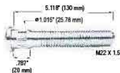
9711-R
