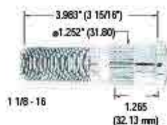
5107-R / 5108-L
