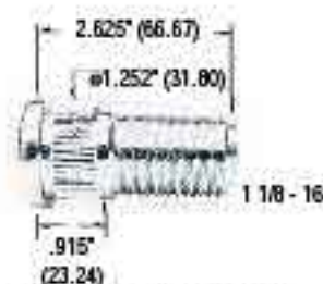
5103-R / 5104-L
