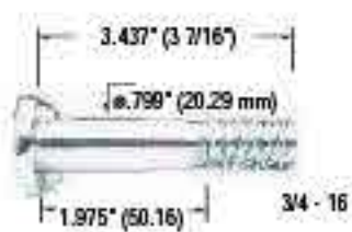
5137-R / 5138-L
