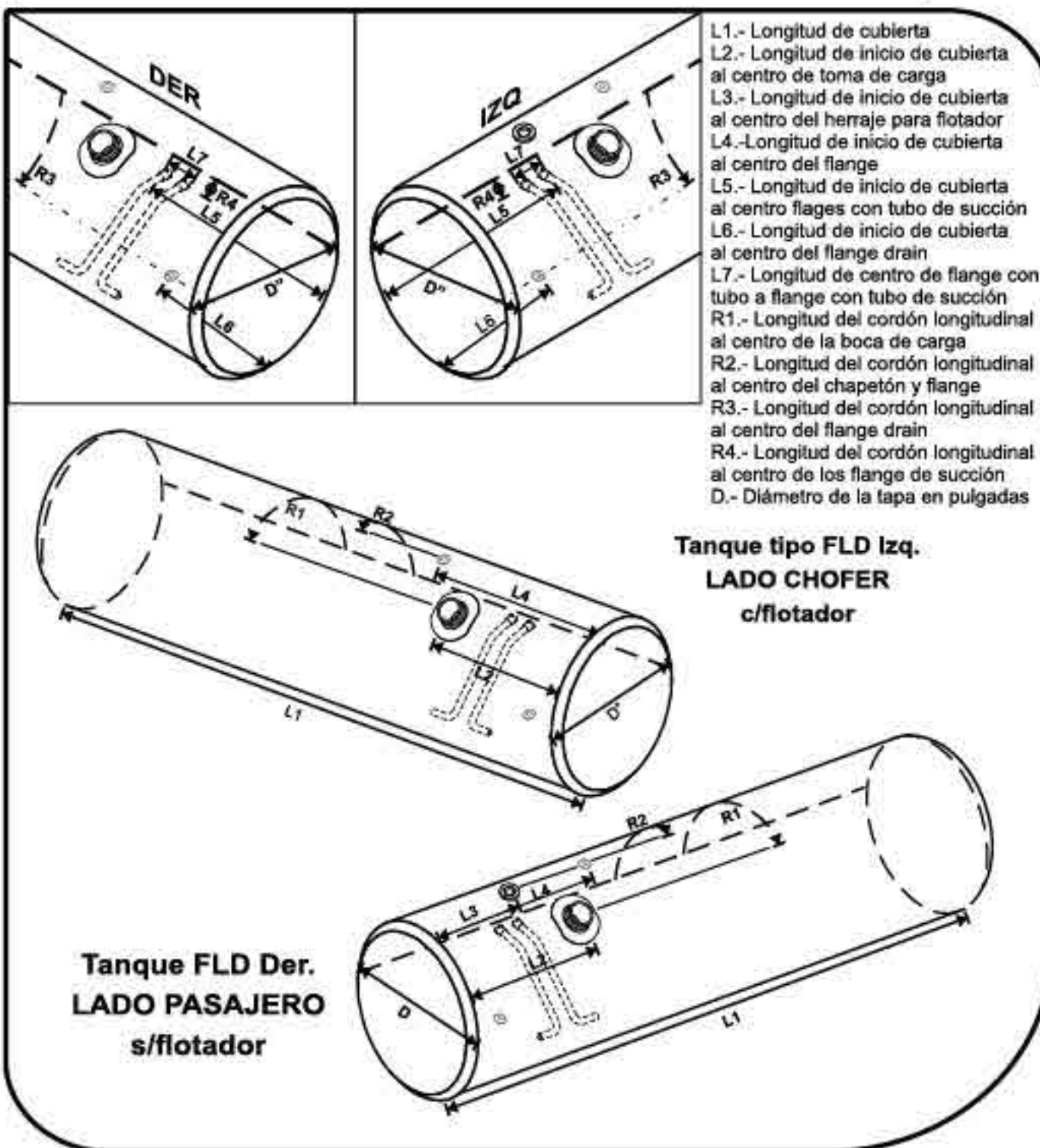
HERRAJE PARA FLOTADOR
