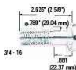
5131-R / 5132-L
