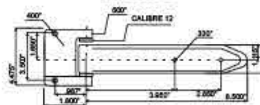
NS-8 NS-8ECO
