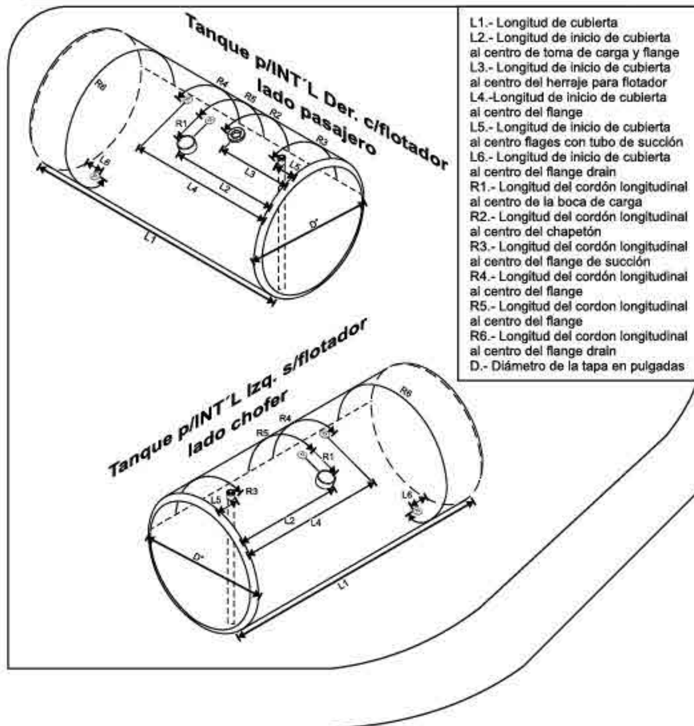
HERRAJE PARA FLOTADOR
