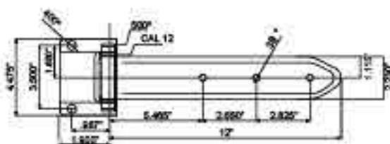
NS-12 NS-12ECO
